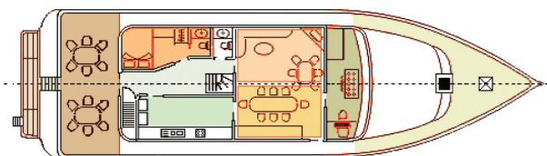
верхняя палуба
